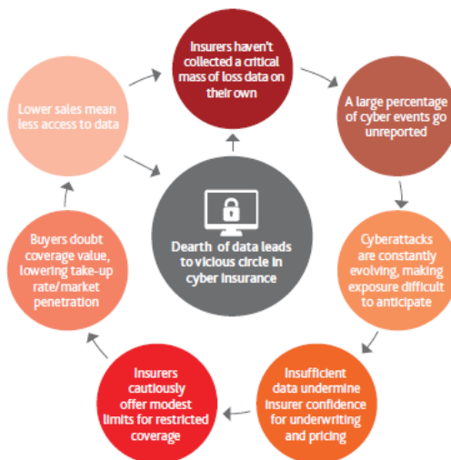
Figura nr. 10. Cercul vicios al asigurărilor ciberneticе
