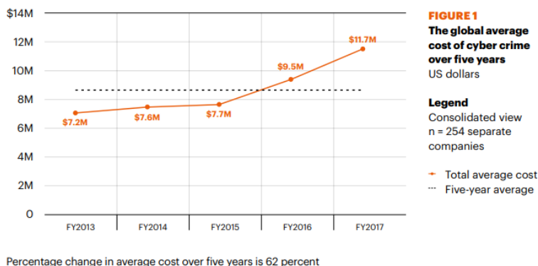
Figura nr. 8. Costul mediu global al criminalității cibernetică în perioada 2013 – 2017
