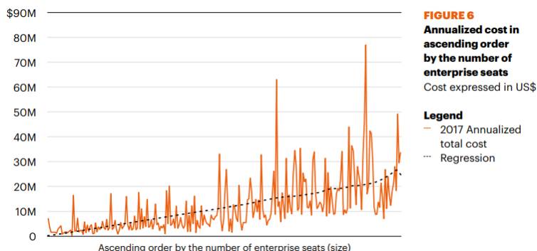
Figura nr. 9. Corelația dintre costul anual al criminalității cibernetice și dimensiunea organizațională a companiilor afectate
