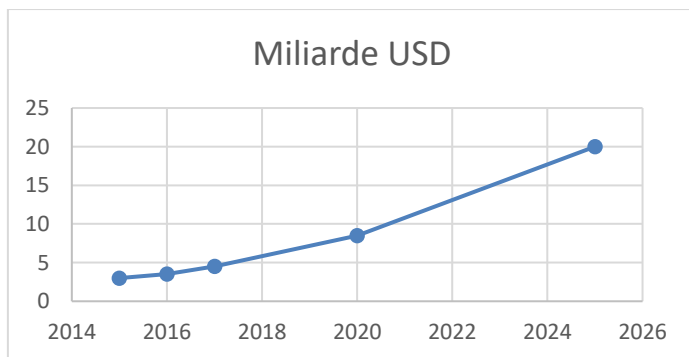
Figura nr. 6. Evoluția primelor subscrise pentru asigurările cibernetic
