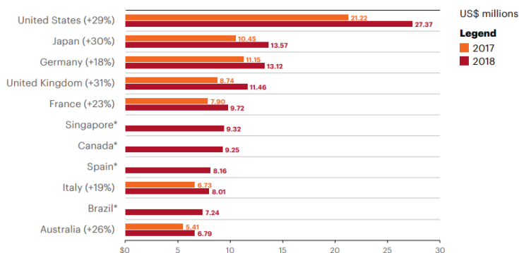
Figura nr. 4. Costurile medii anuale ale crimei cibernetice pe principalele țări afectate
